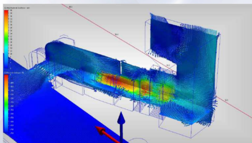
Simulation dynamique d'écoulement
